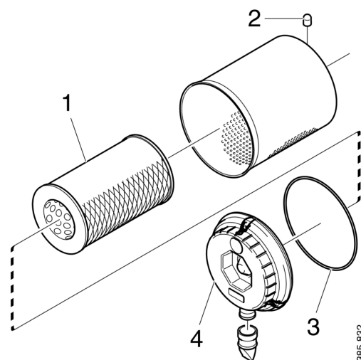
Filtro de ar sem cartucho de segurança:
