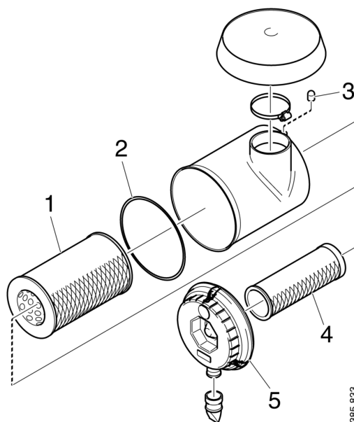
Filtro de ar com cartucho de segurança.
