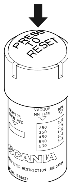
Vacuômetro mecânico com botão de restauração.
