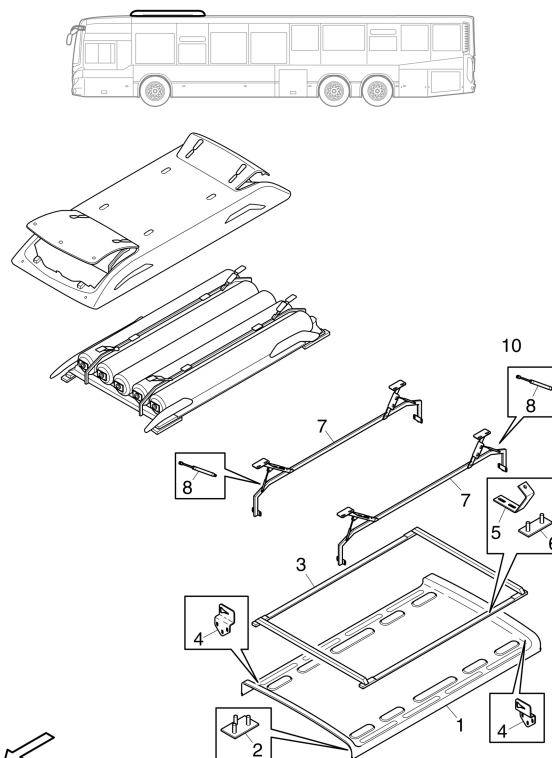
Posição dos pacotes de tanque de gás em ônibus.
