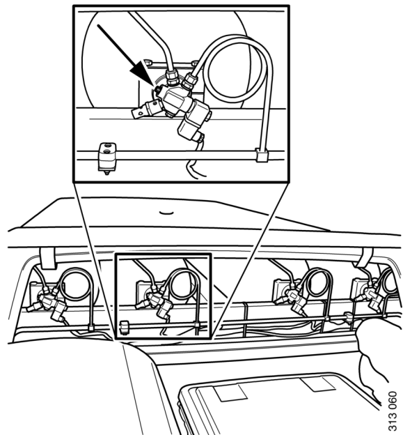
Válvula com interruptor de controle do tanque de gás em ônibus
